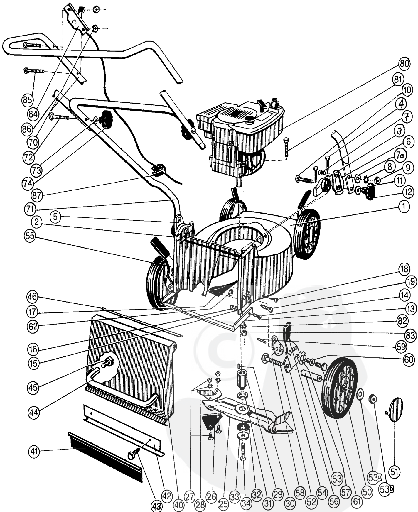
Roto - KING 46 N TYP 1122-01
