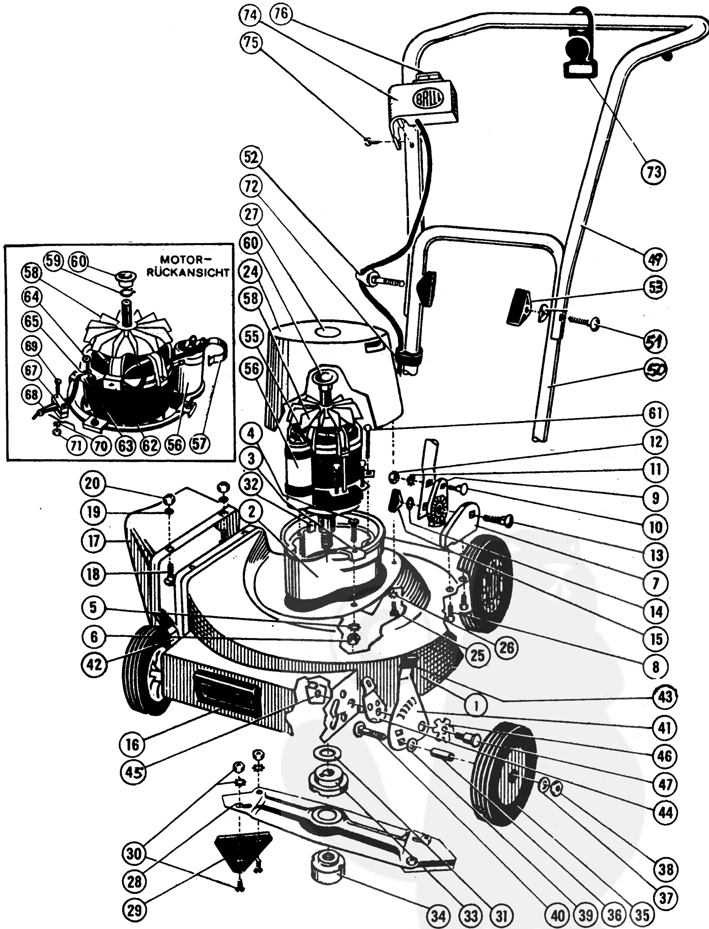
ELEKTRO - FIX 46 TYP 1334
