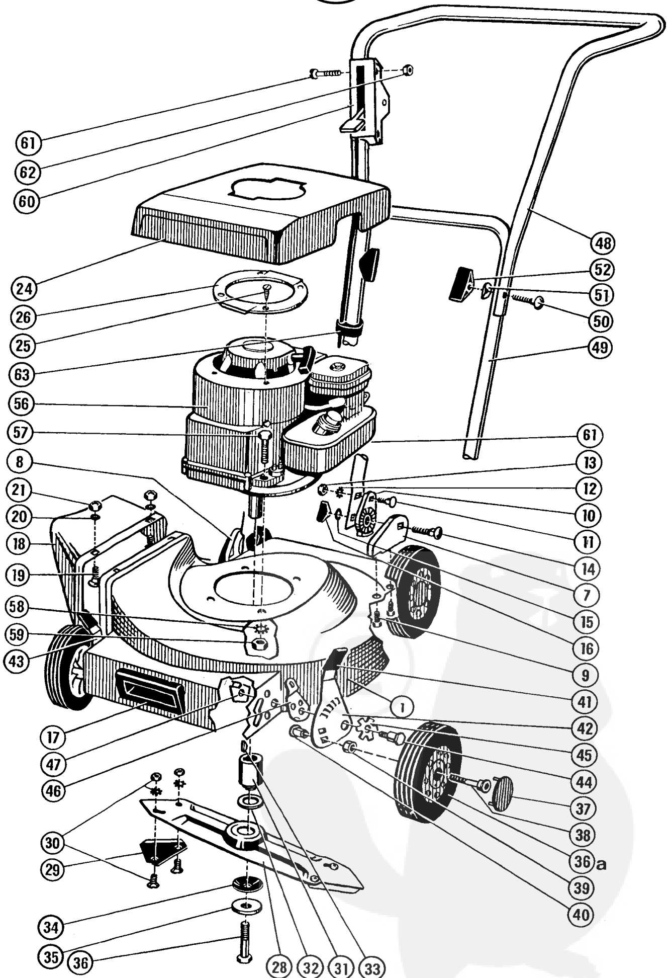
Roto - RAPID 4 TB 46 Typ D (ab S-Nr.930103)
