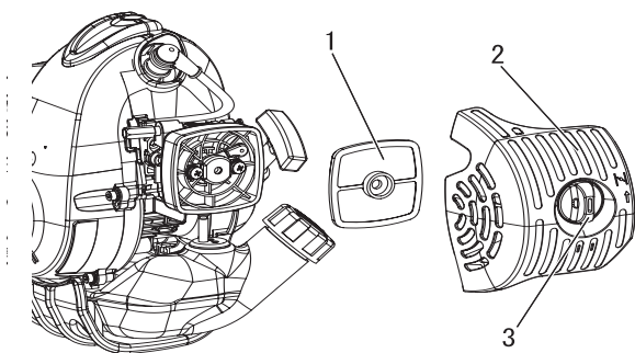
T: Stelschroef voor stationair toerental
