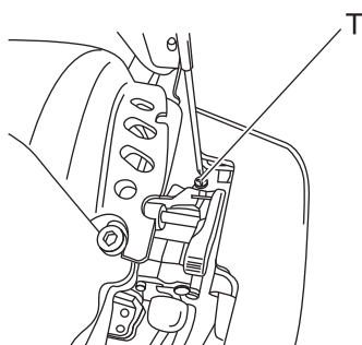
T: Stelschroef voor stationair toerental
