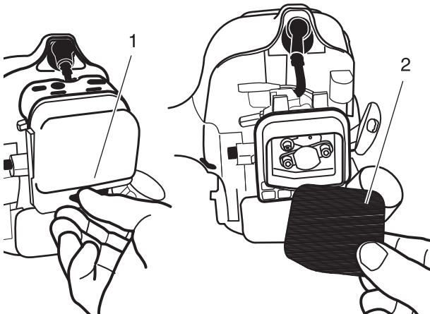
1. Svitare gli elementi di fissaggio 2. Elemento filtrante
