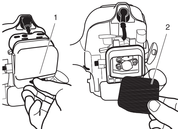
1. Befestigungselemente lösen
