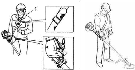
1. Schultergurt
