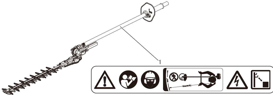
1. Sicherheitsaufkleber (Teilenummer 890617-12361)
