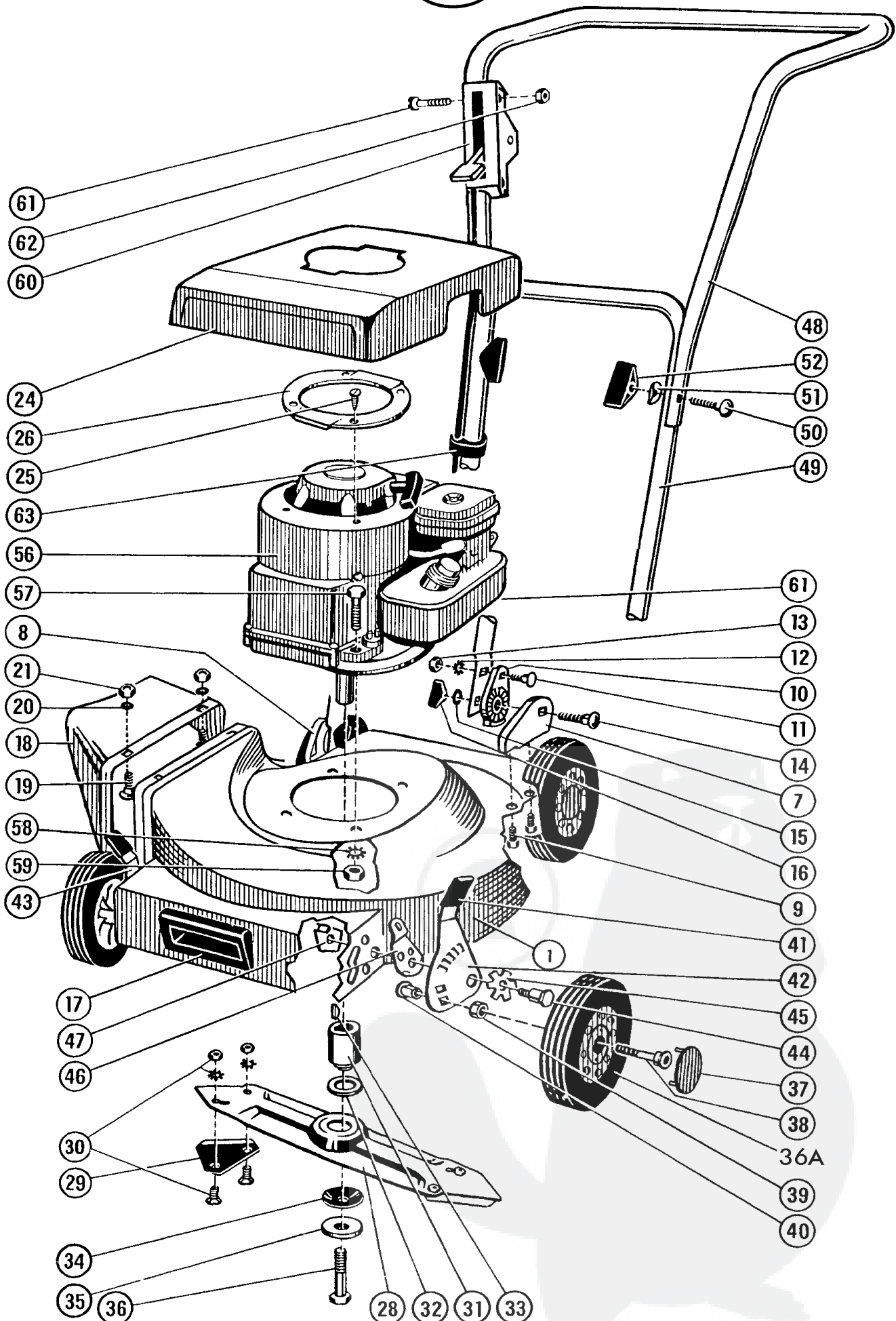
Roto - RAPID 4 TB 46 TYP 0027
