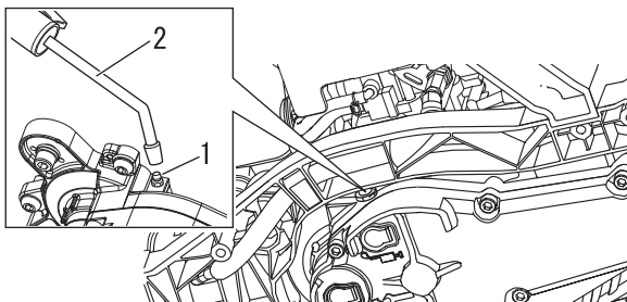
1. Smeernippel
