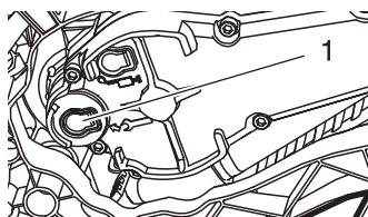
1. Pakkingring
