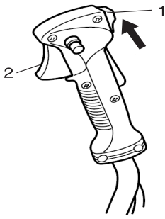
1. Ontstekingsschakelaar 2. Handgastrekker
