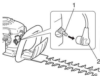
2. Bougiekabel
