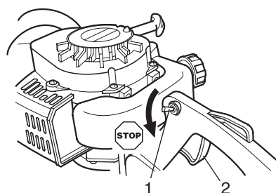
1. Ontstekingsschakelaar 2. Handgastrekker
