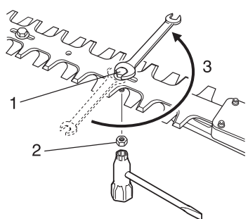
3. 1/2 slag losdraaien
