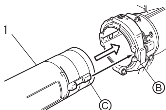
1. Blazerbuis (hoofdbuis)
