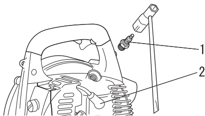
2. Bougiekap
