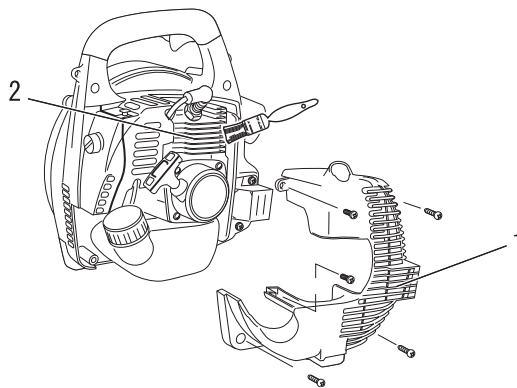
1. Motorafdekking
