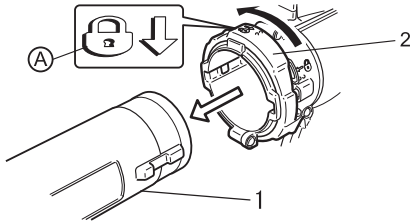
1. Tuyau de soufflage (tuyau droit)
