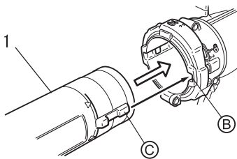
1. Tubo del soplador (tubo recto)
