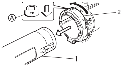
1. Rohr (gerades Rohr)
