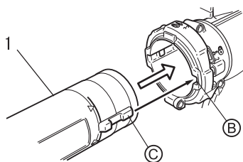
1. Condotto del ventilatore (condotto dritto)
