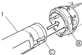
1. Rohr (gerades Rohr)
