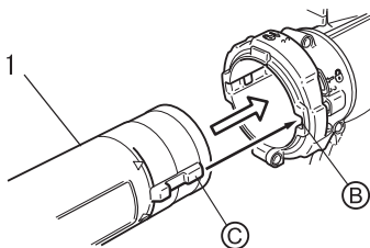
1. Tuyau de soufflage (tuyau droit)
