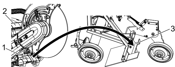
1. Beschermplaat 2. Snijzaag 3. Montageplaatje voor voorste handgreep
