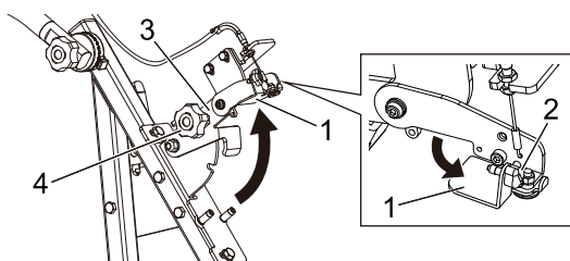
1. Gasklepplaatje 2. Knop van gasklepplaatje 3. Plaatje van achterste handgreep 4. Zaagvergrendelknop
