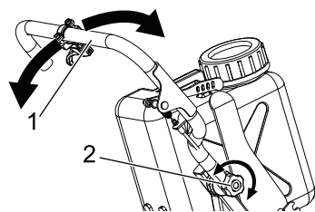
1. Handgreep van wagen 2. Handgreepvergrendelknop
