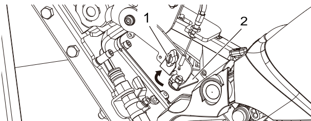
1. Knop van gasklepplaatje 2. Gasklepplaatje
