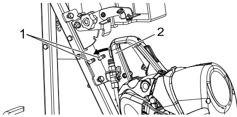
1. Geleidepennen 2. Achterste handgreep
