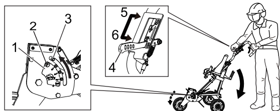
1. Diepteafstellingsplaatje 2. Ruststand 3. Diepteafstellingsindicator 4. Hendel voor diepteafstelling 5. Vrije zijde 6. Vergrendelde zijde
