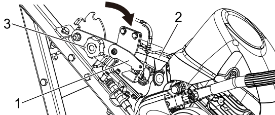
1. Plaatje van achterste handgreep 3. Zaagvergrendelknop 2. Achterste handgreep
