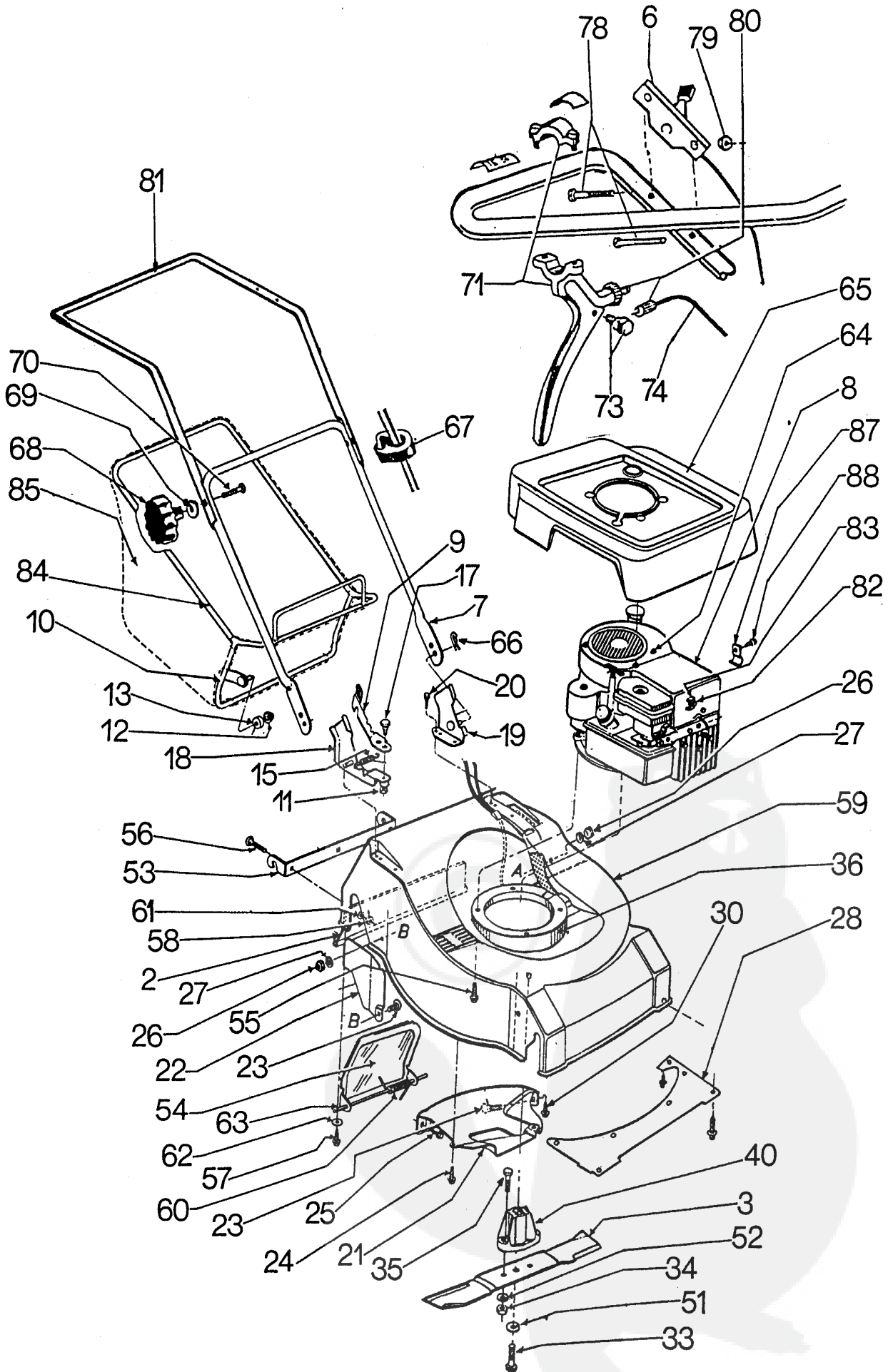
Roto - MONARCH 56 TYP 2151-01
