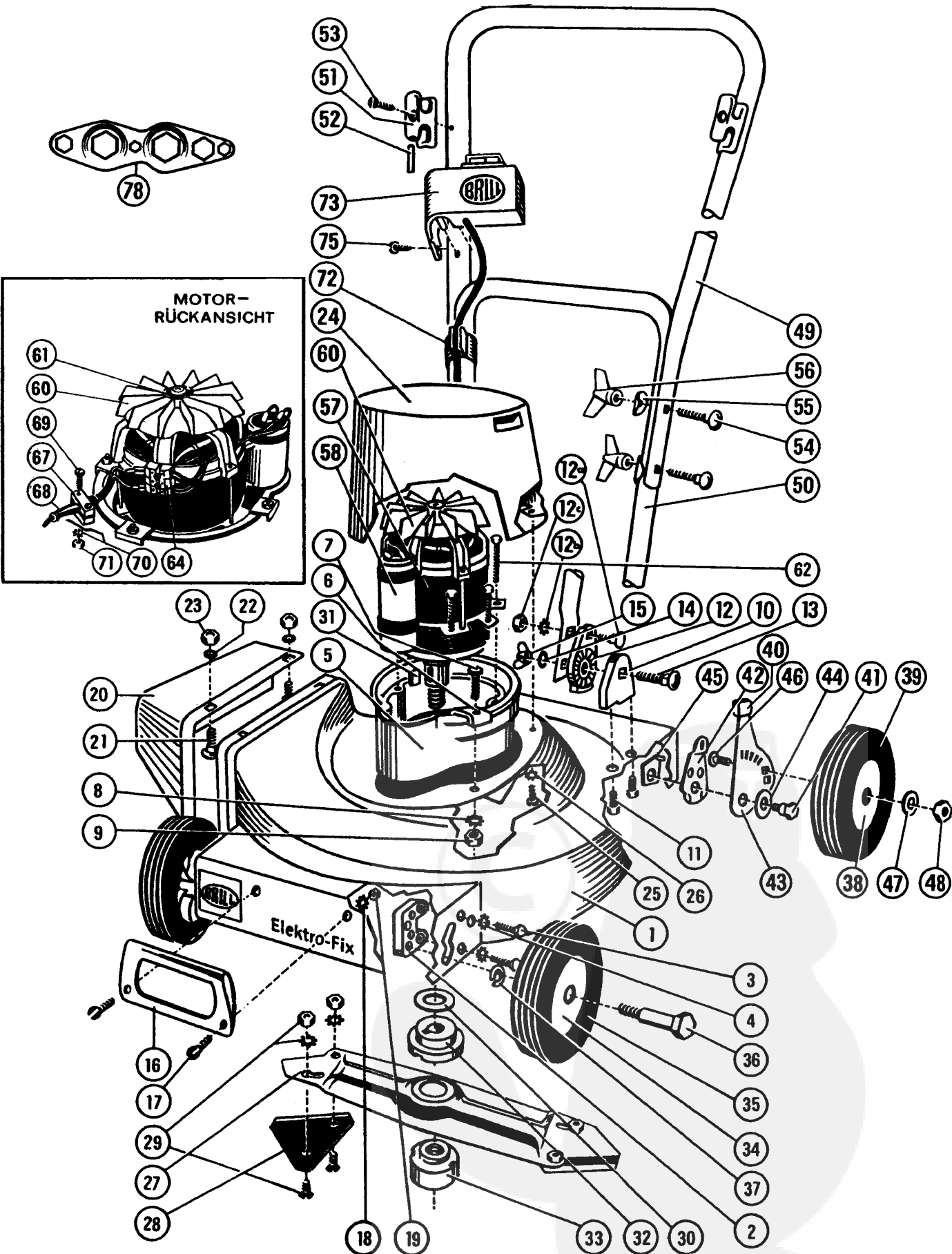
ELEKTRO - FIX 46 TYP F
