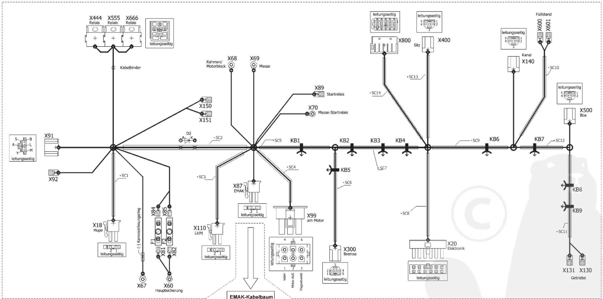
EMAK-Kabelbaum 473661 6170-440-0500-A
